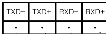
CNV485NS 녹색커넥터 단자
